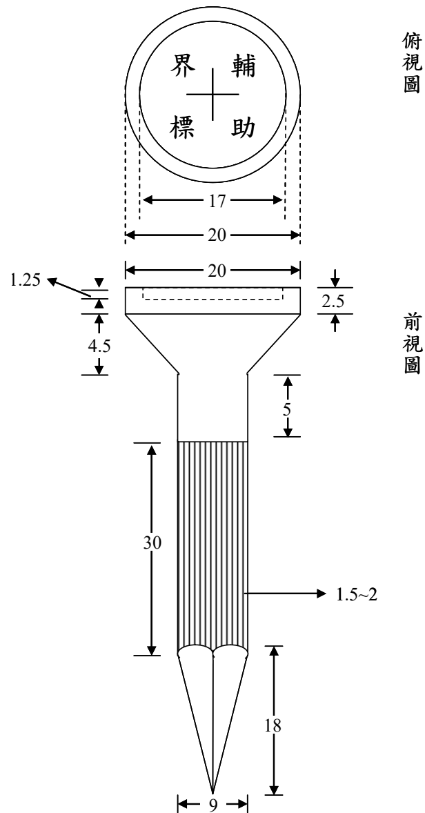
鋼釘界標（輔助界標）
