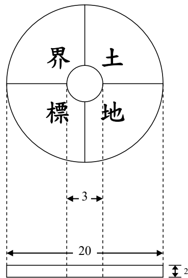
鋼釘界標（土地界標）
