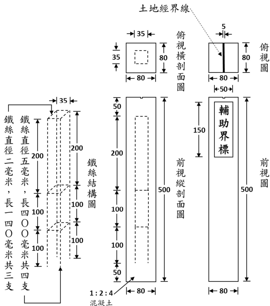
水泥界標（輔助界標）
