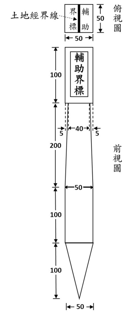
塑膠界標（輔助界標）
