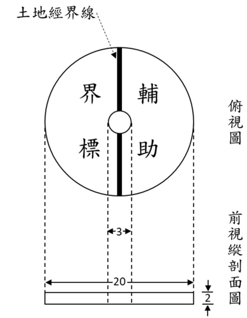
鋼釘界標（輔助界標）
